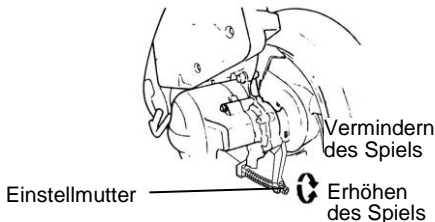
Hinterrad-Trommelbremse
