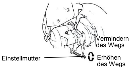
Hinterrad-Trommelbremse
